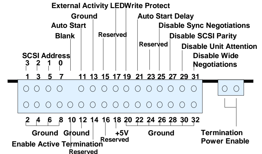
Dimensionamento dei ponticelli (vista frontale) - Tutti i modelli. * Non disponibile per il Mod. 80 Pin SCA
